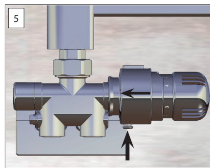
Poussez la bague de verrouillage vers la vanne et appuyez sur le bouton de verrouillage
