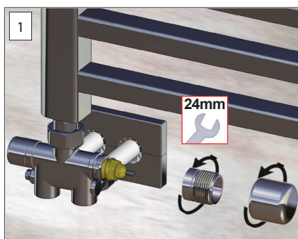
Dévisser la poignée et le support fileté de la vanne, à l'aide d'une clé de 24 mm
